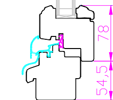
RUSTIKAL profiil
